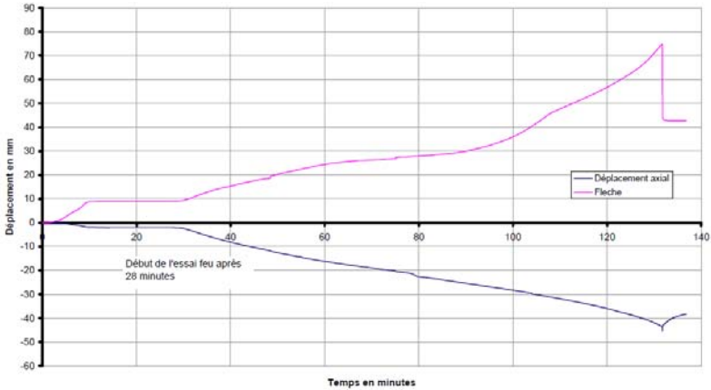
Déplacements mesurés par les capteurs de déplacement
