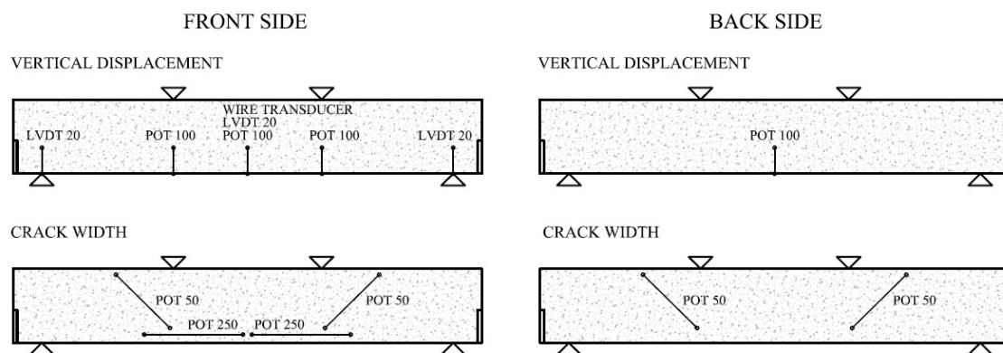
Figura 2 : Strumentazione
