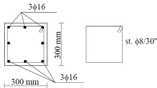
Figura 9: Geometria della sezione analizzata
