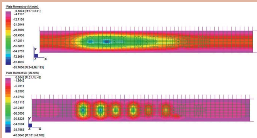
13a - Momenti in direzione x ed y nel caso di non diffusione del carico.
