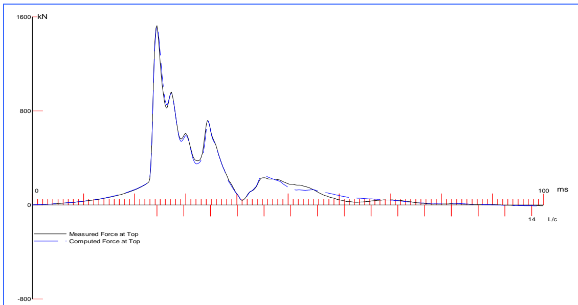
Diagramma forza – tempo
