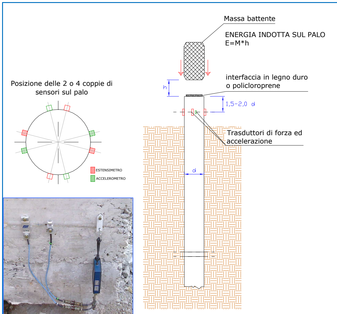
Schema della prova Case
