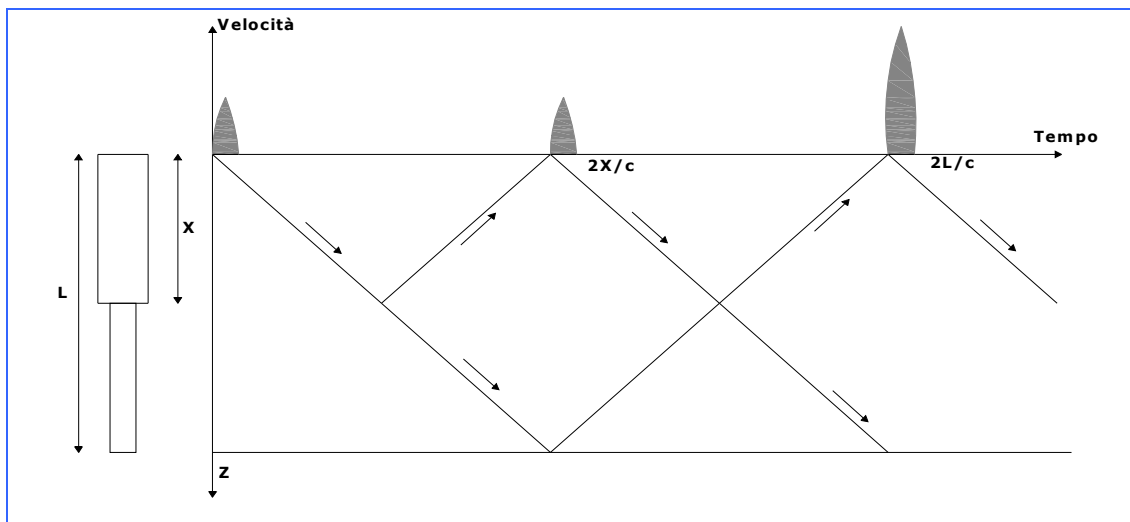
Esempio di riflessione dell'onda dovuto ad un difetto
