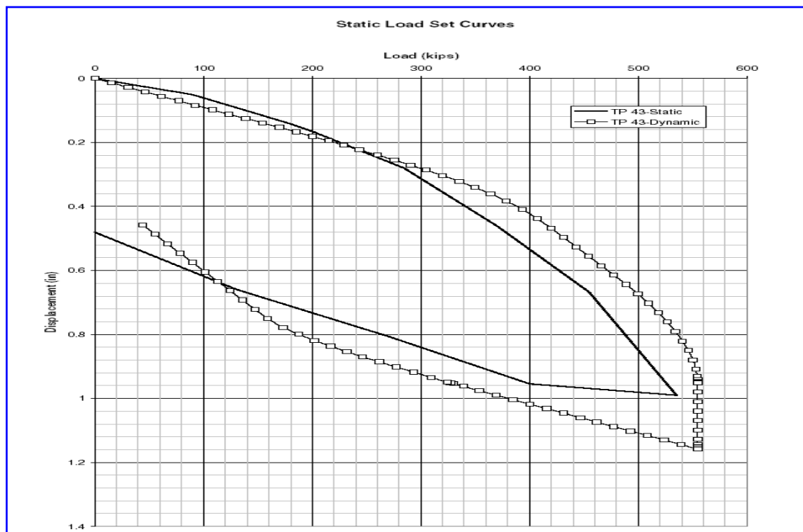
Confronto dei diagrammi carico - cedimento
