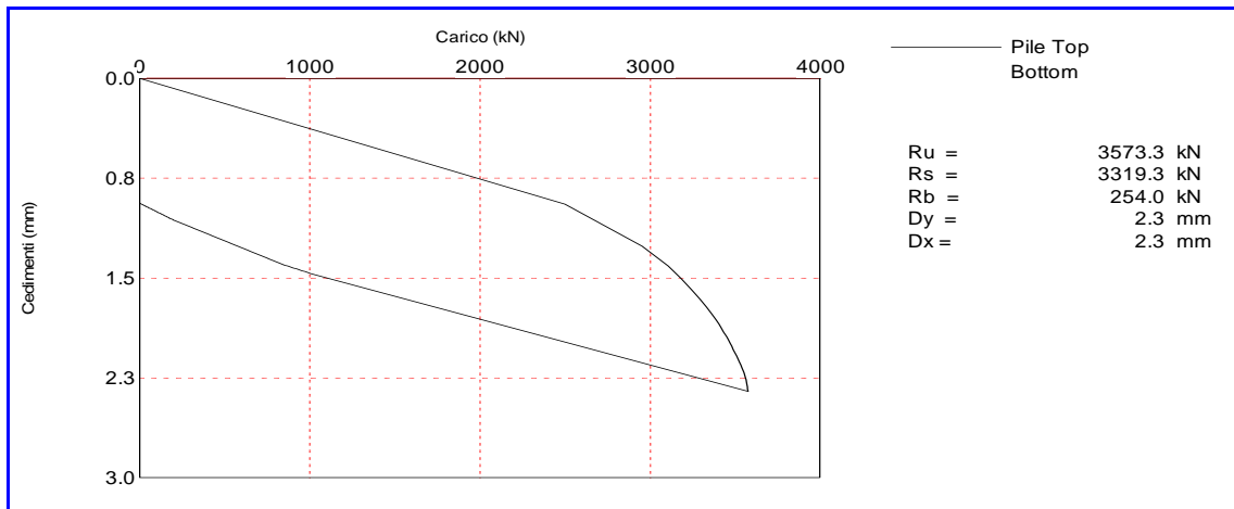
Diagramma carico - cedimento
