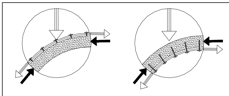
Figura 4. Dettaglio dell'interfaccia tra tirante e muratura. (a sinistra) cavo estradossale con connettori in compressione (a destra) cavo intradossale con connettori in trazione
