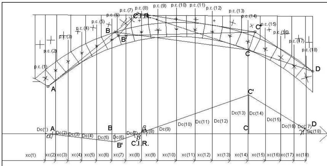
Figura 26. Peso dei conci e componente verticale dello spostamento virtuale
