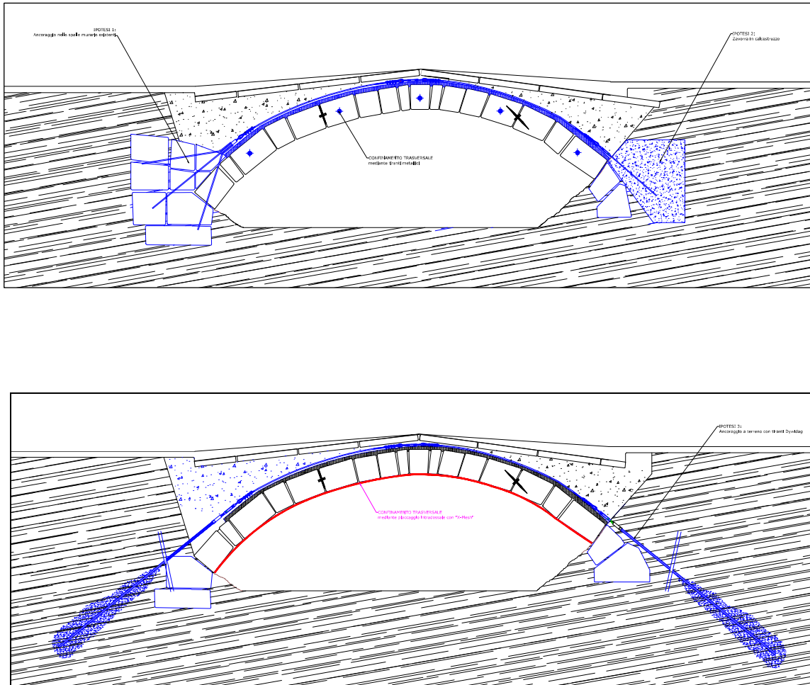
Figura 39. Ipotesi di intervento formulate in funzione della consistenza delle zone di imposta
