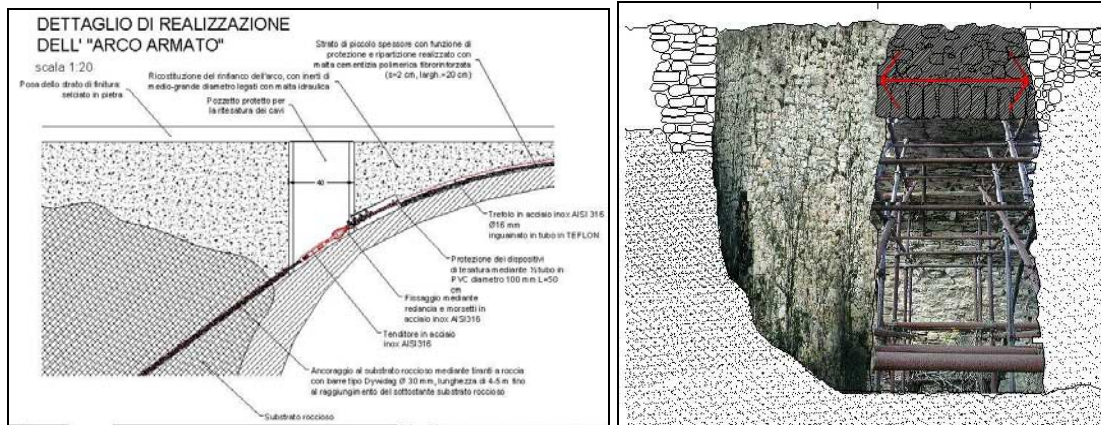
Figura 31. schema degli interventi di consolidamento statico
