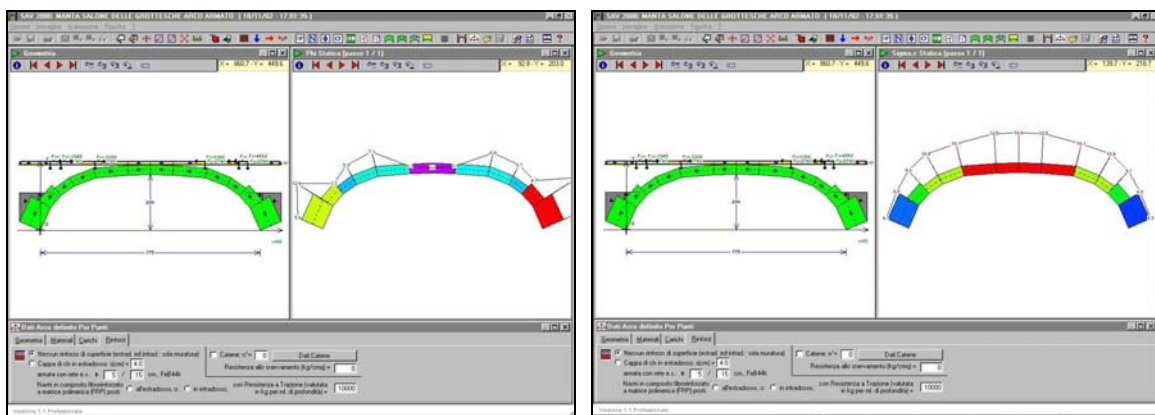
Figura 21. Programma SAV 2000: OUTPUT GRAFICI - grafico degli sforzi di scorrimento tra i conci e grafico degli sforzi normali ai conci
