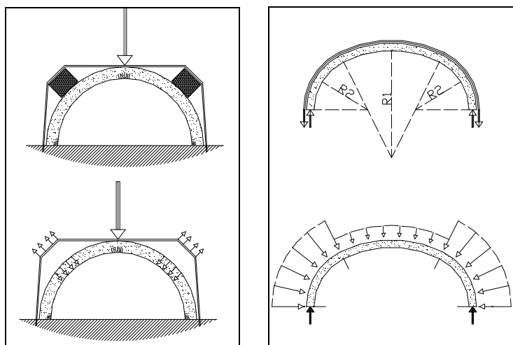
Figura 5. (a sinistra) "Forzatura" localizzata tra arco e tirante di estradosso per opporsi a imbozzamenti locali. (a destra) Si noti che le forze dipendono dal raggio di curvatura locale applicate dal cavo teso all'arco
