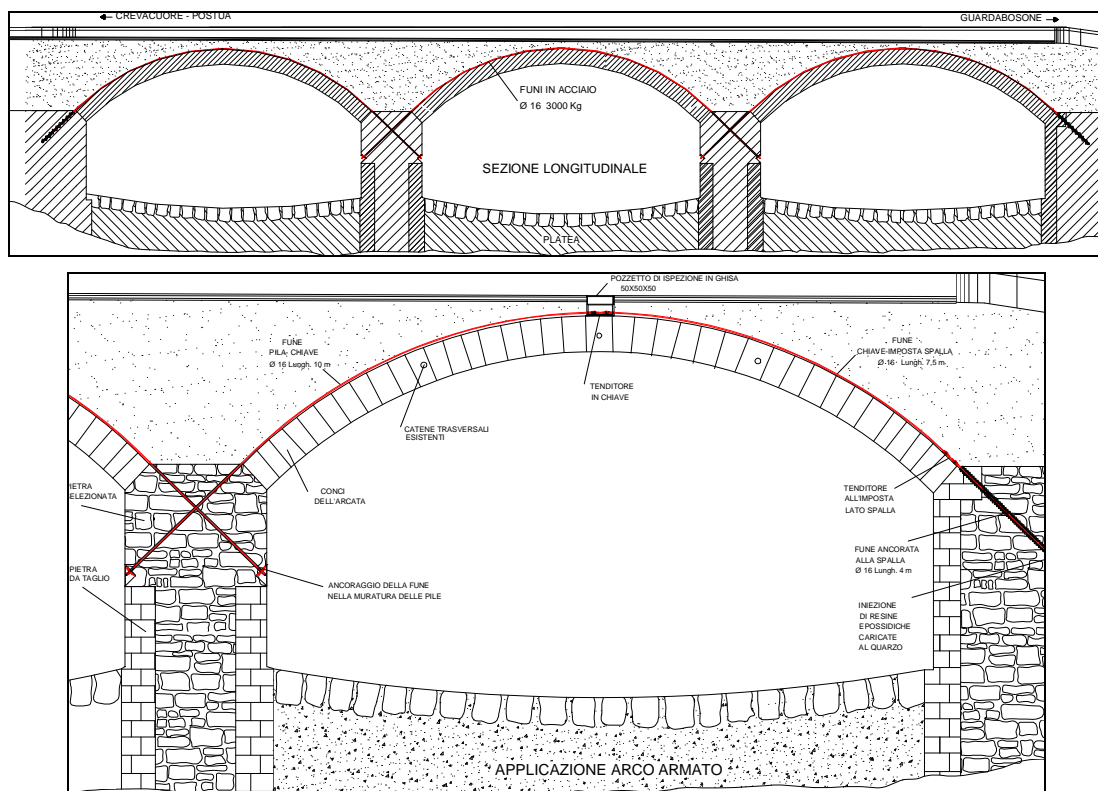
Figura 24. Elaborati di progetto.
