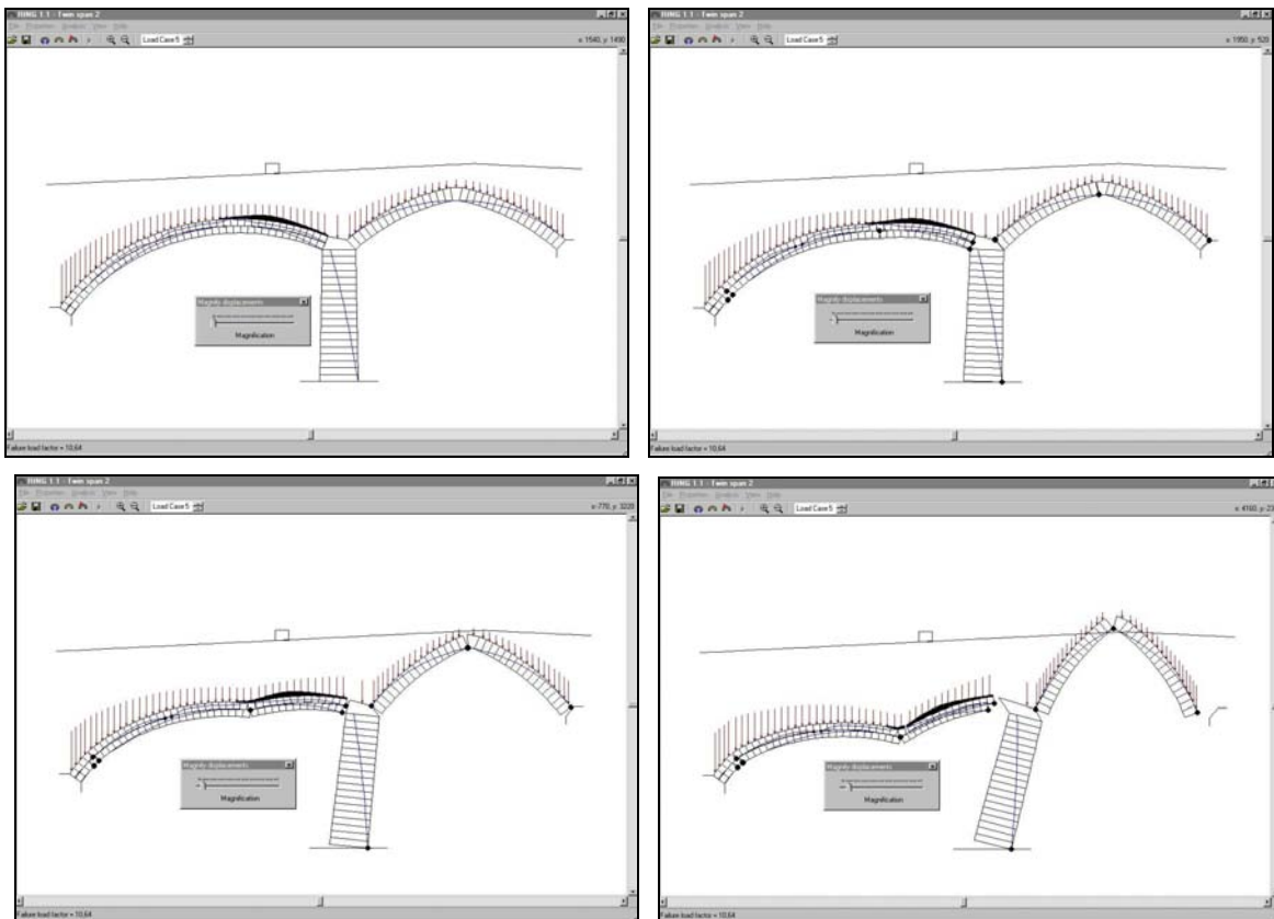
Figura 16. Programma Ring : es.1 - cinematismo di rottura
