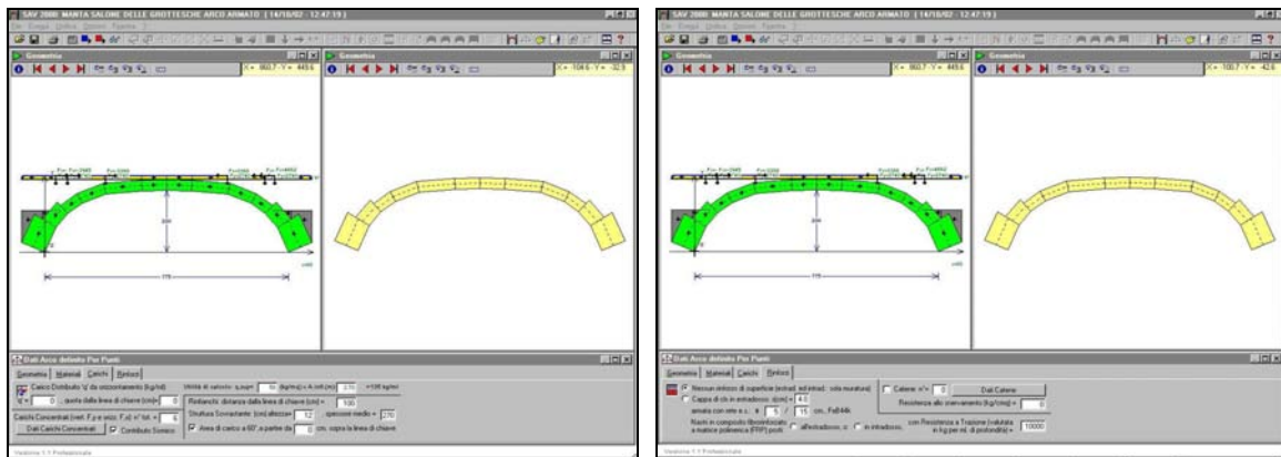
Figura 19. Programma SAV 2000: introduzione dei carichi e introduzione di catene e rinforzi.
