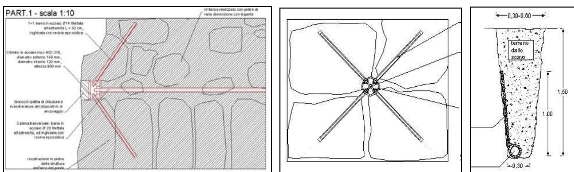
Figura 32. Particolari di progetto.
