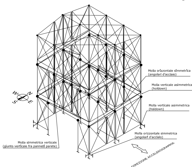
Figura 13. Modello numerico dell'edificio provato.
