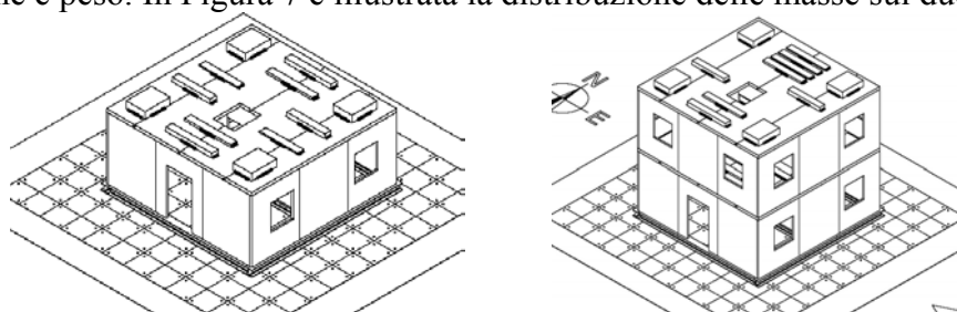
Figura 7. Distribuzione delle masse d'acciaio al primo e secondo piano.
