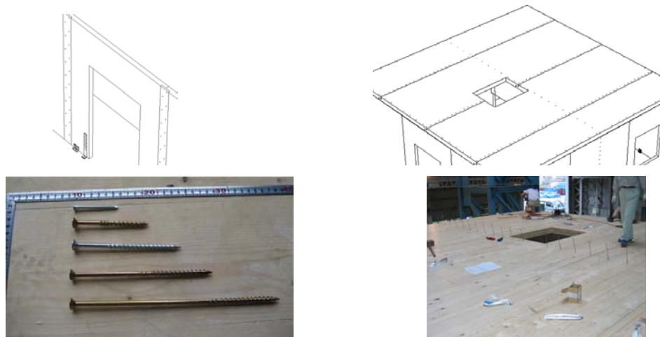
Figura 5. Giunti verticali tra i pannelli parete e giunti orizzontali tra i pannelli solaio e viti autoforanti utilizzate per i collegamenti.
