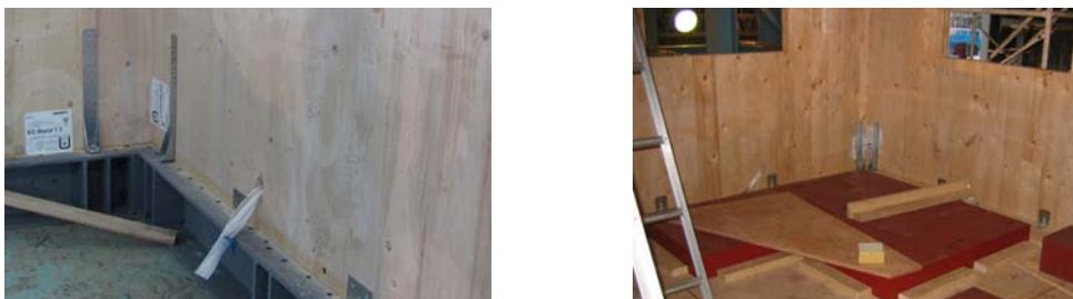
Figura 6. Collegamento delle pareti al piano terra e al piano primo con holdown e angolari d'acciaio.
