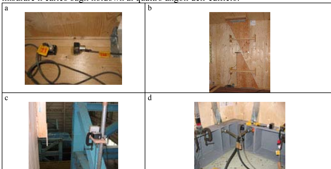
Figura 8. Strumenti diversi utilizzati nelle prove: a , accelerometri; b , dispositivo per la misurazione dello spostamento interpiano; c , trasduttore a filo; d , celle di carico a rondella.
